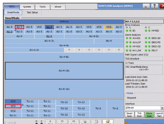
FTB-8115 SmartMode: 使用实时告警扫描发现多通道信号（显示在FTB-500用户界面中）
