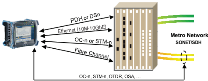
FTB-500平台具有模块化、多插槽的设计结构，允许用户根据其测试需求在现场升级系统，从而节省投资
