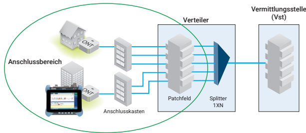
Abbildung 1: Zertifizierung des FTTx-Anschlussbereichs mit Splitter-Durchgang
