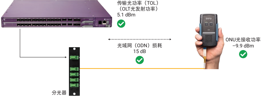
图1: 光功率读数
