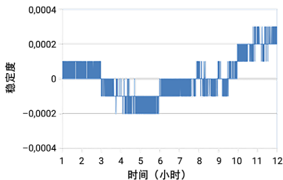
图2: 12小时内的功率稳定性
