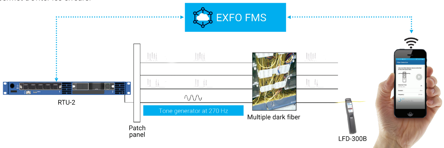
Figure 3. Mode source/tonalité pour l'identification des fibres.
