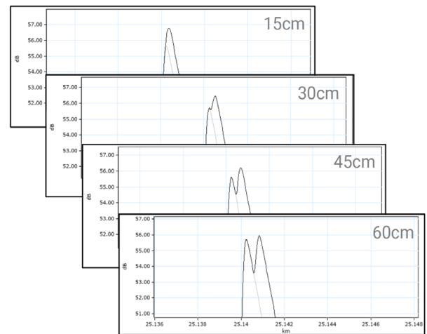
Figure 1. Démarcation haute résolution des ports de terminaison PON à l'aide de HRD jusqu'à 60 cm.
