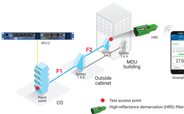
Figure 2. Certification des liaisons dans une architecture PON avec connectivité de bout en bout.
